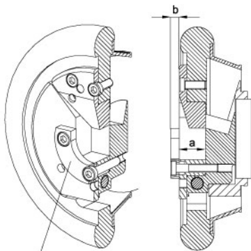
軸向定位環
