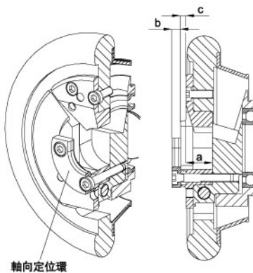
軸向定位環
