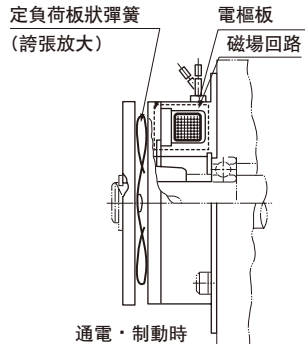
制動器動作
