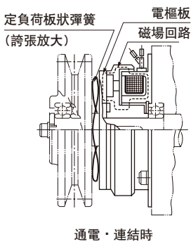
離合器動作
