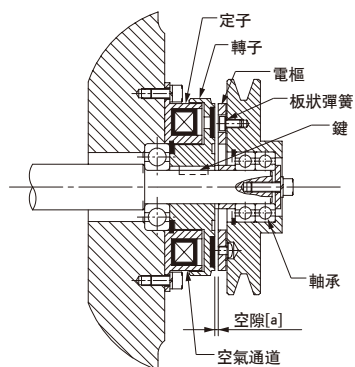
法蘭安裝型構造 (FCD機型)
