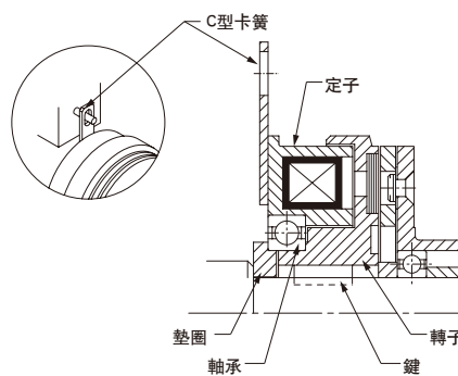
定子·轉子的安裝 (軸承安裝型)
