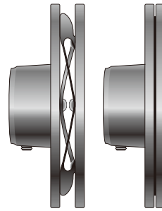
板狀彈簧的動作
