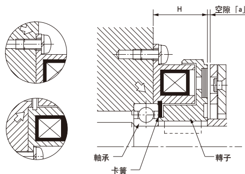
定子·轉子的安裝 (法蘭安裝型)
